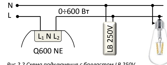
Рис 2.2 Схема подключения с балластом LB 250V
