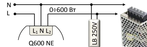
Рис 2.4 Универсальная схема подключения Q600 NE
