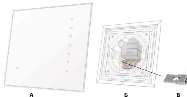
Рис 1 Состав выключателя светорегулирующего Q600 NE
