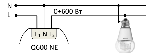
Рис 2.2 Схема трехпроводного (с N-проводом) подключения
