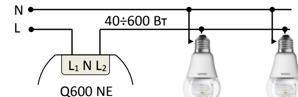
Рис 2.1 Основная схема подключения Q600 NE (двухпроводная)
